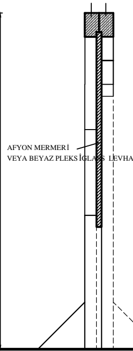
B-B KESİTİ
